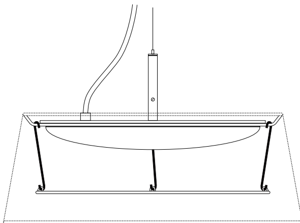
Querschnitt / cross-section
